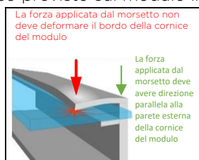
Figura 1 Forza applicata dal morsetto
